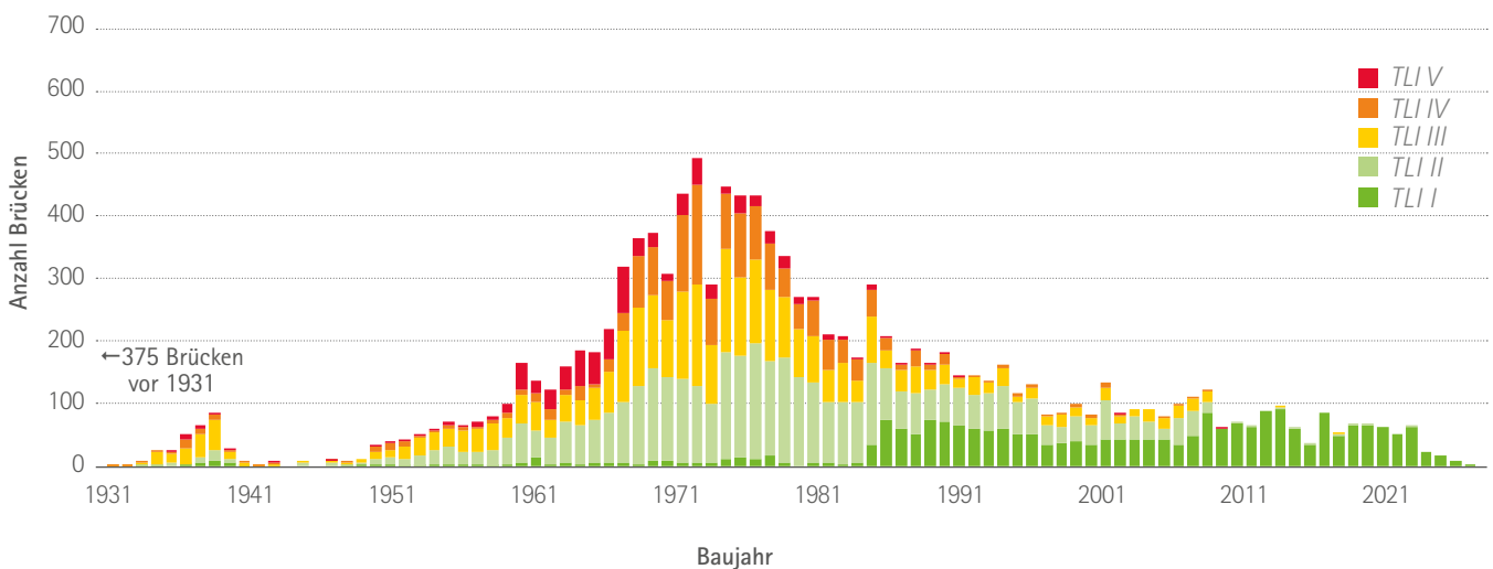
Abbildung 3: Bitte ändern in: Altersstruktur der Brücken nach Traglastindex I - V (Bund und Land)
